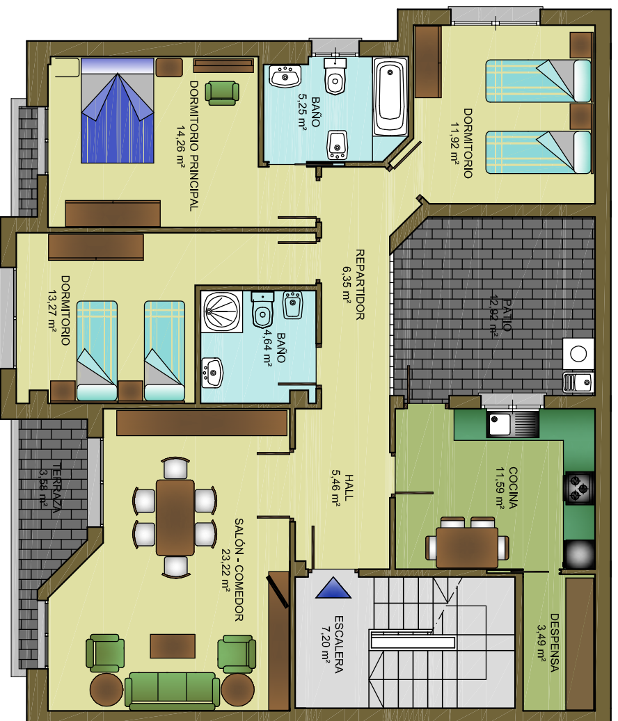
PLANTA PRIMERA
